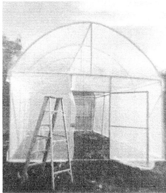
โรงเรือนปลูกพืชหลังคาโค้ง ขาตรงแบบเคลื่อนที่ได้ ขนาด ๔ x ๘ เมตร
